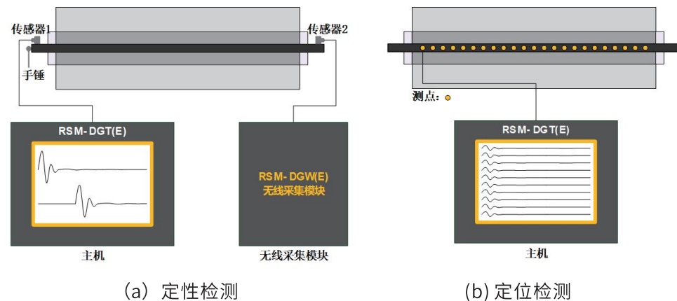
图3-1 桥梁孔道灌浆质量检测仪基本原理
