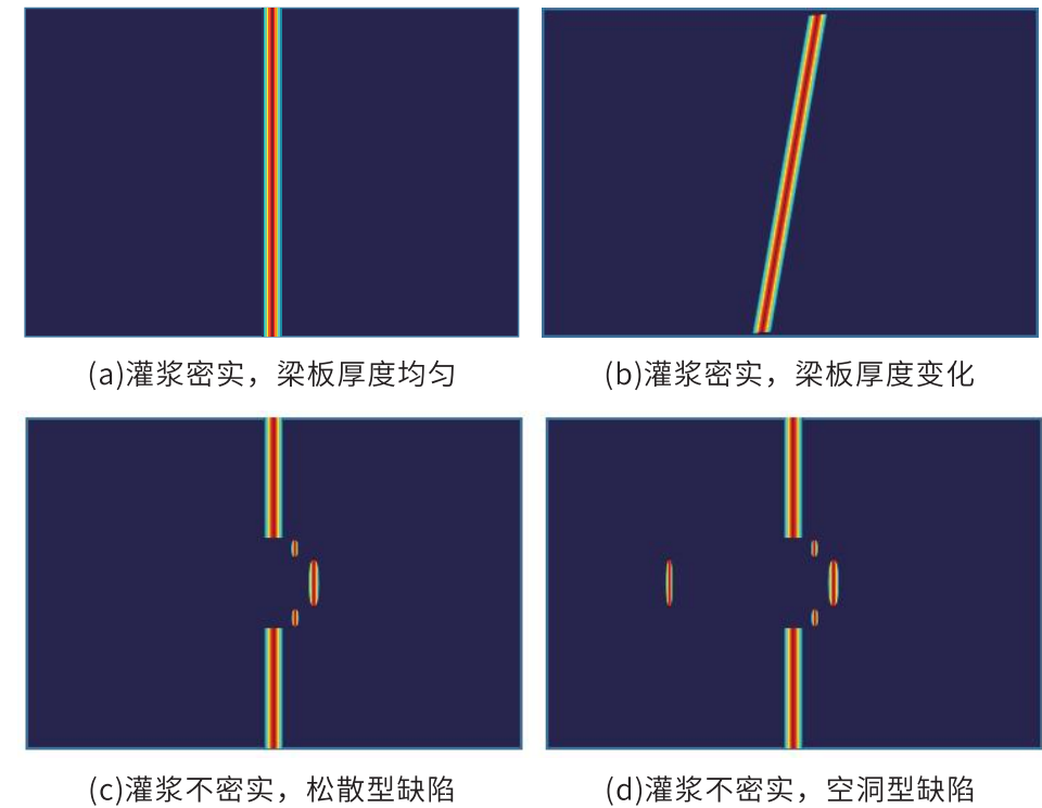
图3-5 定位检测色谱图参考
