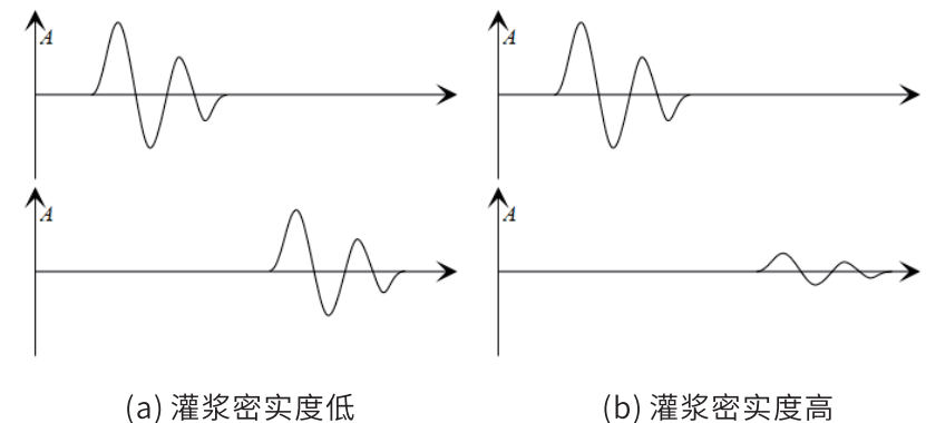
图3-3 全长衰减法示意图
