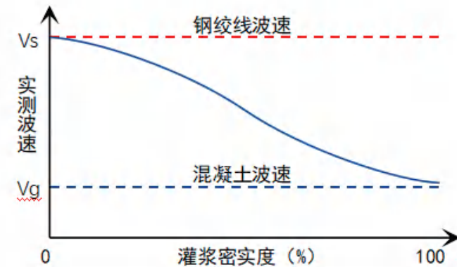
图3-2 全长波速法示意图
