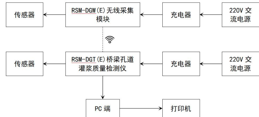
图2-3 RSM-DGT(E)桥梁孔道灌浆质量检测仪检测外围设备示意图
