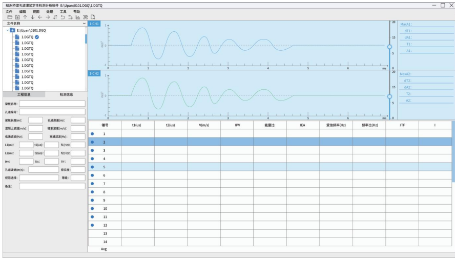
图5-8 批量分析视图
